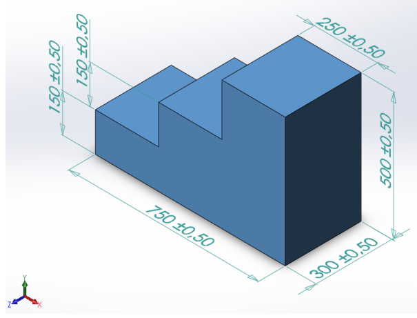
Şekil-8 Görev 1 Malzemelerinin Yerleştirileceği Alan Ölçüleri (İzometrik Görünüm)
