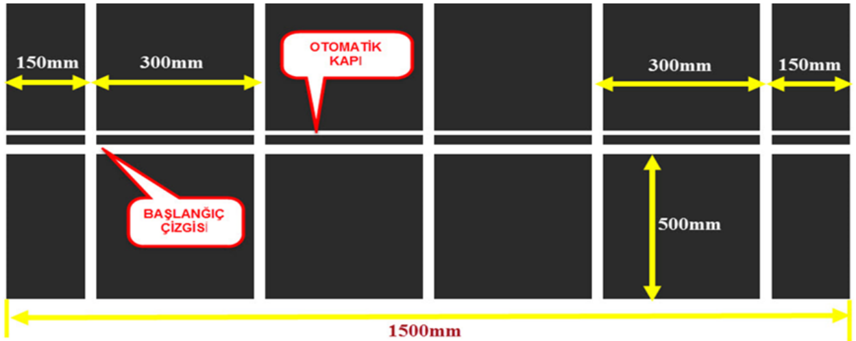
Şekil-1: Hızlı Çizgi İzleyen pisti ölçüleri
