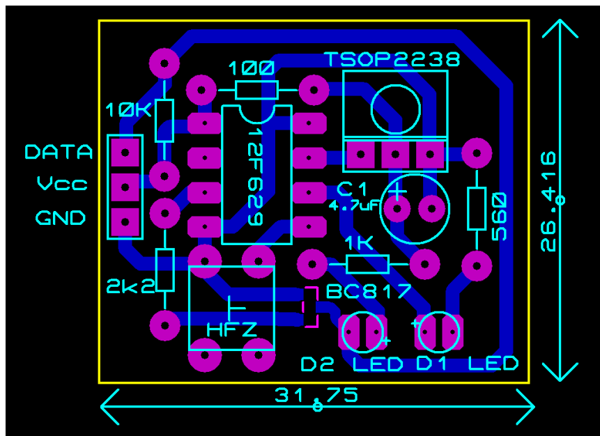
Şekil 2 : Start Module PCB
