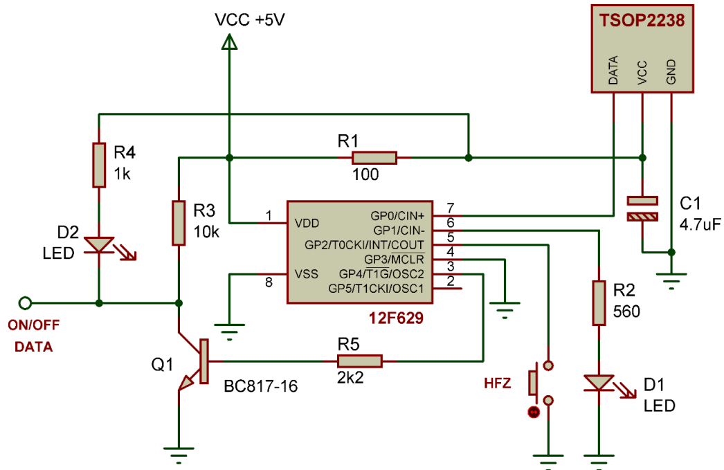
Şekil 1 : Start Module circuit
